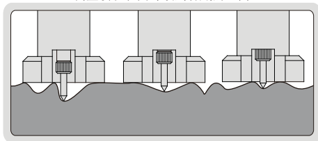
测量喷砂表面峰顶到谷底的距离
